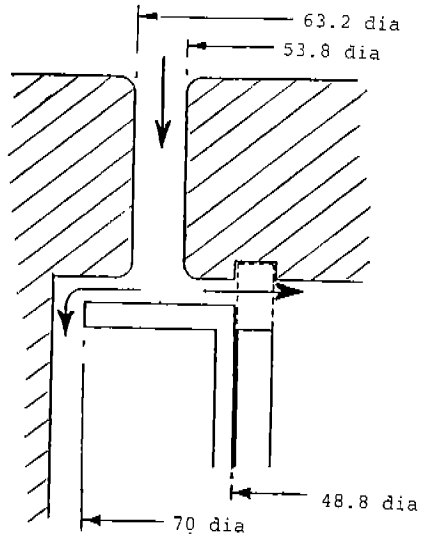
FIGURE 2 RING VALVE (D) PORT-PLATE SECTION. (all sizes mm)
